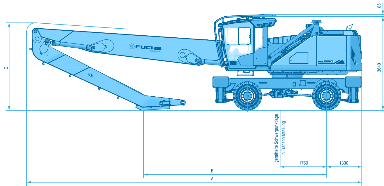
SEITENANSICHT (alle Maße in mm)
