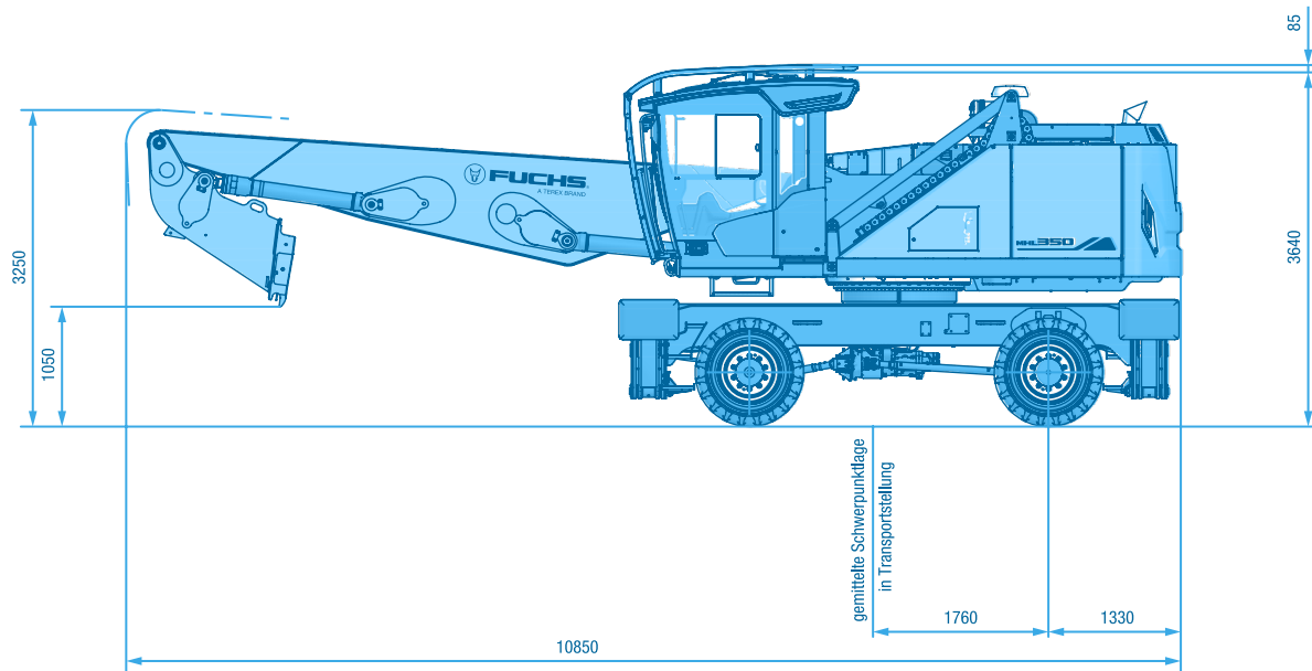
SEITENANSICHT FQC (alle Maße in mm)
