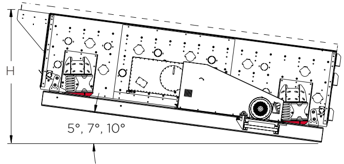
5°, 7°, 10° Wedges
